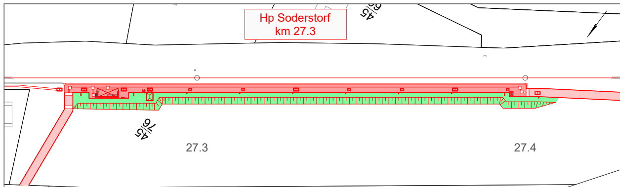
Lageplan des zukünftigen Bahnhofs
